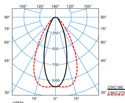
7651IP MironaF T 200-840ET L150 01ESG (LEO1)
