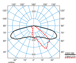
Publisca P3-AB2L-MLLR/16-42-730 4G1 ETDD (CLO end value)
