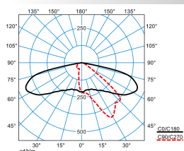
Publisca P3-AB2L-MLLR/16-42-730 4G1 ETDD (CLO initial value)
