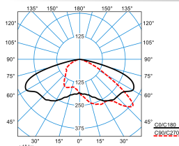
LnPlus 40-AB7L-LR/15000-740 12G1 ET (CLO initial value)
