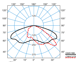
LnPlus 40-AB7L-LR/15000-740 12G1 ET (CLO end value)
