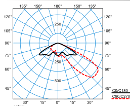
LnPlus 60-AM19L-LR/20000-727 16G1 ET (CLO initial value)
