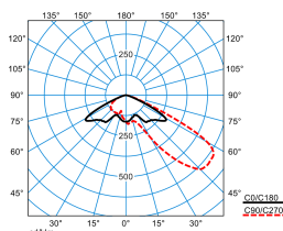
LnPlus 60-AM19L-LR/20000-727 16G1 ET (CLO end value)
