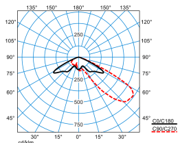
LnPlus 70-AM19L-LR/38000-730 36G1 ET (CLO end value)
