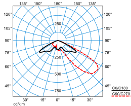
LnPlus 70-AM19L-LR/38000-730 36G1 ET (CLO initial value)
