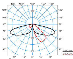
8841LS-UE 260-AB2L/3200-740 3G2 ET (CLO end value)
