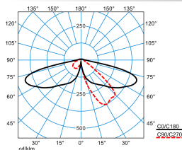
8841LS-UE 260-AB2L/3200-740 3G2 ET (CLO initial value)
