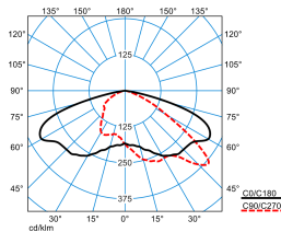
LnPlus 40-AB7L-LR/6200-730 6G1 ET (CLO initial value)
