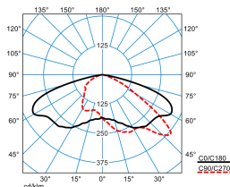
LnPlus 40-AB7L-LR/15000-727 12G1 ET (CLO end value)
