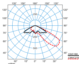
LnPlus 40-AM19L-LR/2200-722 2G1 ET (CLO end value)
