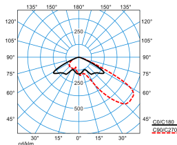
LnPlus 40-AM19L-LR/2200-722 2G1 ET (CLO initial value)
