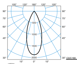
Altigo G2 10 RB17L/300-830 1G1P + VE IP66 24V DC 80W
